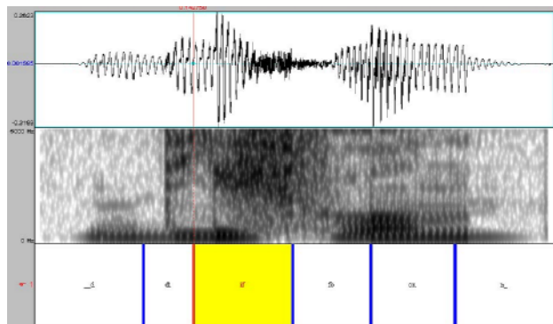
Rys.1 Proces segmentacji
